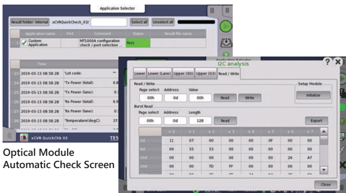
Optical-Module Check
